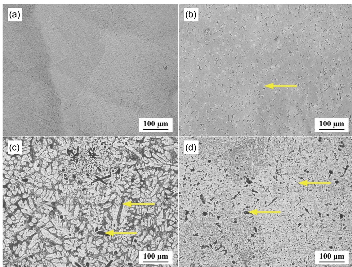
Fig. 3: Optical microstructure of solution-treated alloys: (a) TE0, (b) TE1, (c) TE2 (d) TE3
